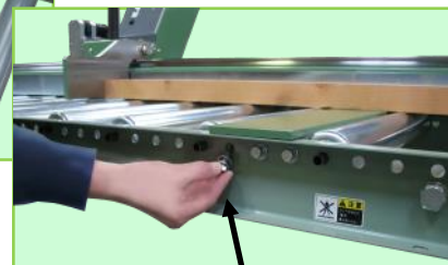
既存のコンベアにボルトで固定
